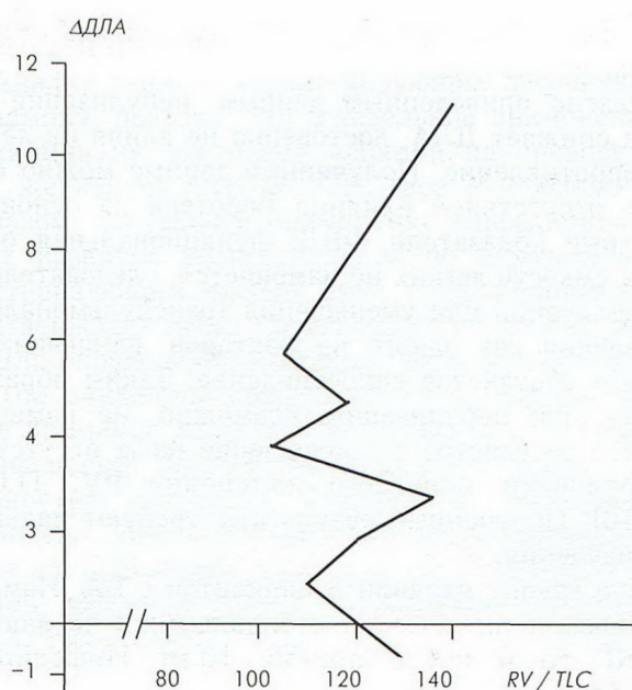
Рис. 1. Криволинейная корреляция
