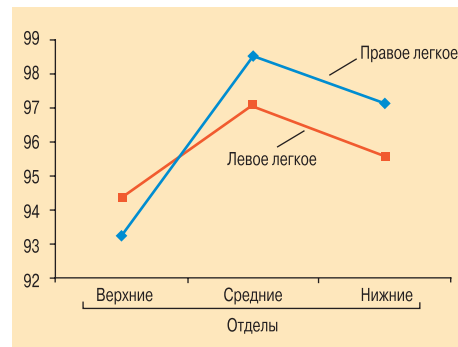
Рис. 2. Изменения средних значений градиентов плотности легочной ткани в правом и левом легком у пациентов с ДСТ
